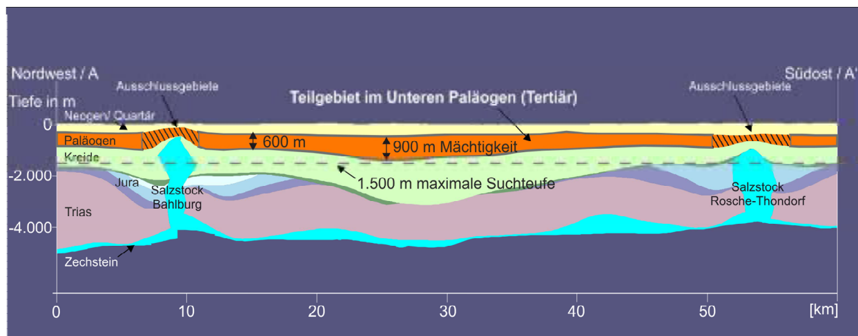
Abbildung 6: Geologischer Profilschnitt durch das Teilgebiet 004_00TG_053_00IG_T_f_tpg (überhöhte Darstellung)
