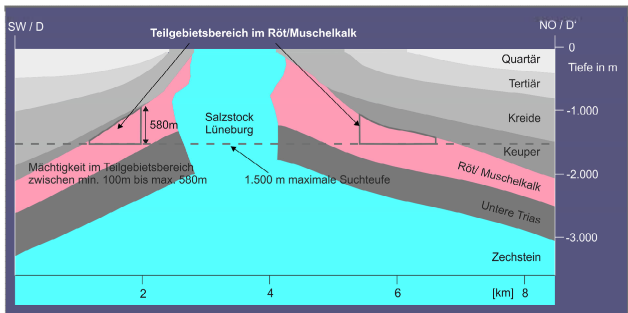
Abbildung 41: Geologischer Profilschnitt durch den Teilgebietsbereich 076_02TG_191_02IG_S_f_so
