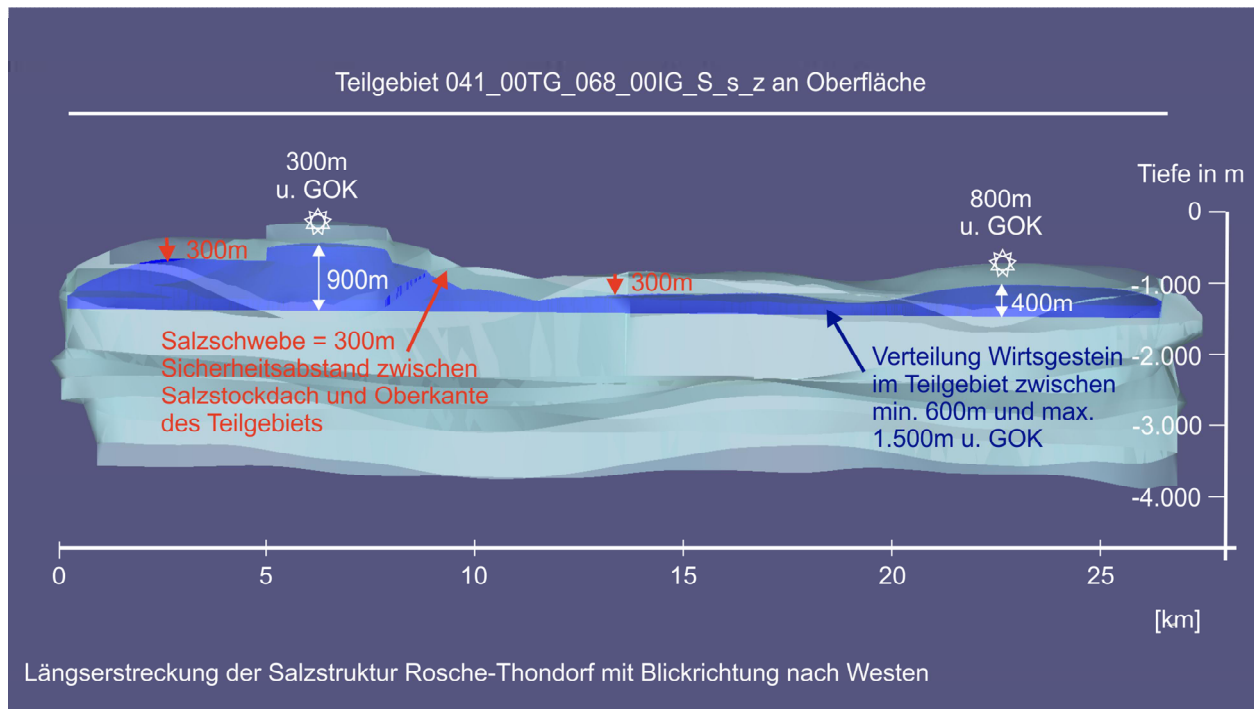
Abbildung 34: Perspektivische Darstellung des Teilgebiets 041_00TG_068_00IG_S_s_z im Salzstock Rosche-Thondorf
