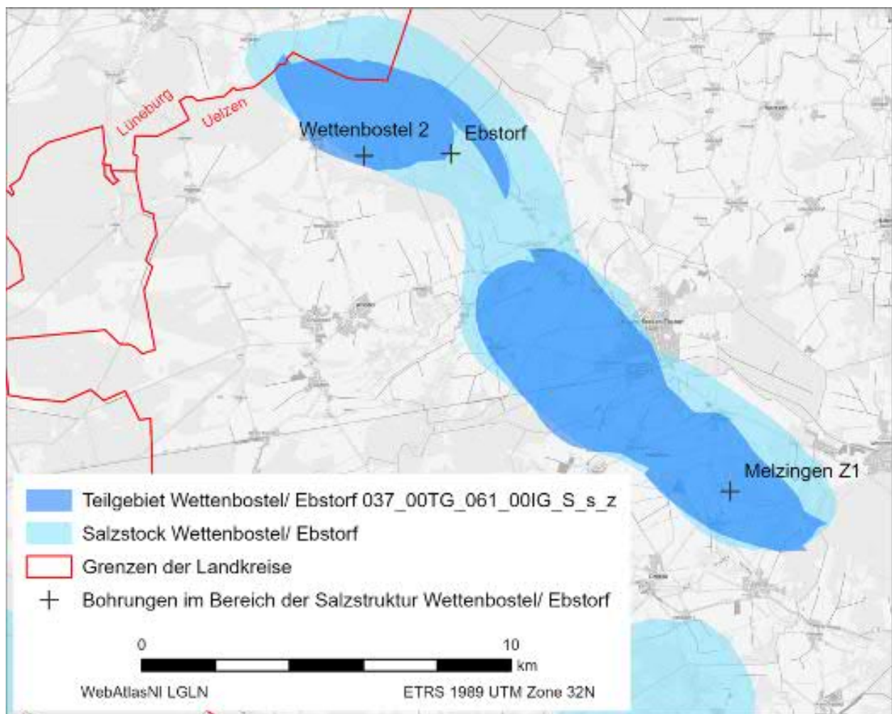
Abbildung 21: Übersichtskarte des Teilgebiets 037_00TG_061_00IG_S_s_z
