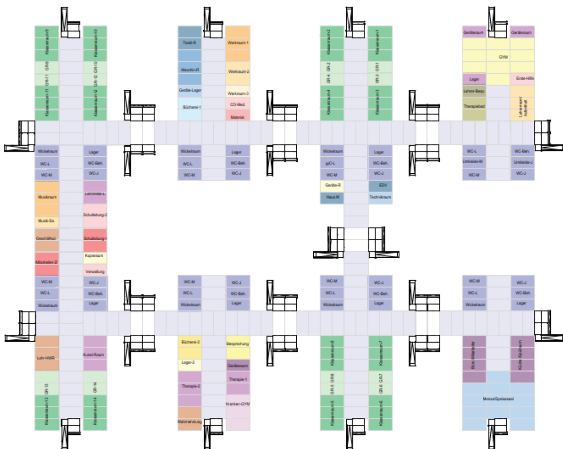
Abbildung 28 – Ausschnitt Konzeptplanung Fa. Adapteo, Anlage 5c
